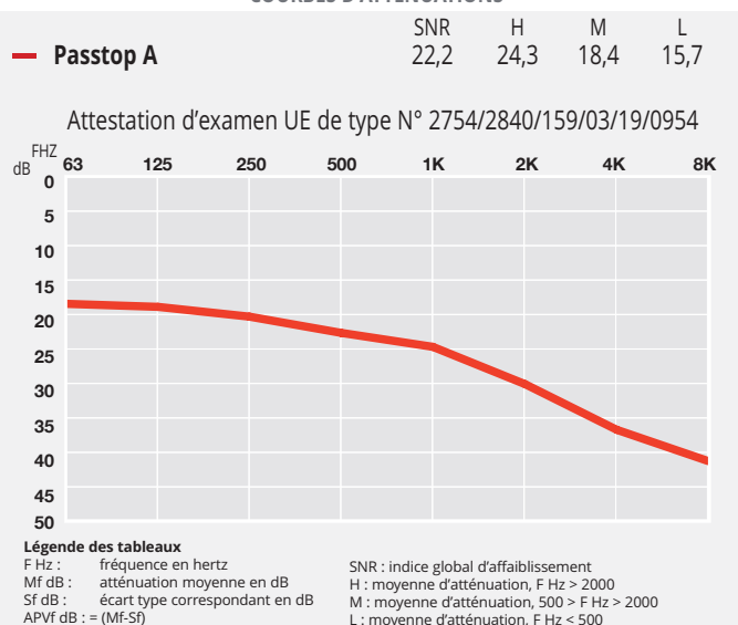
COURBES D'ATTENUATIONS
